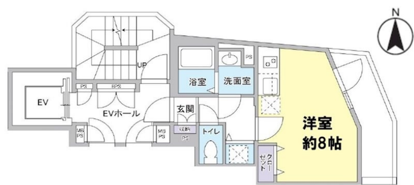
【間取り図】
