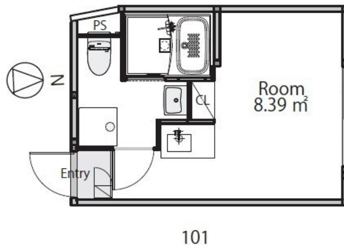
【間取り図】
