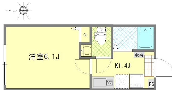
【間取り図】
